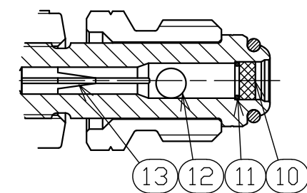
B 詳細(1:1)
